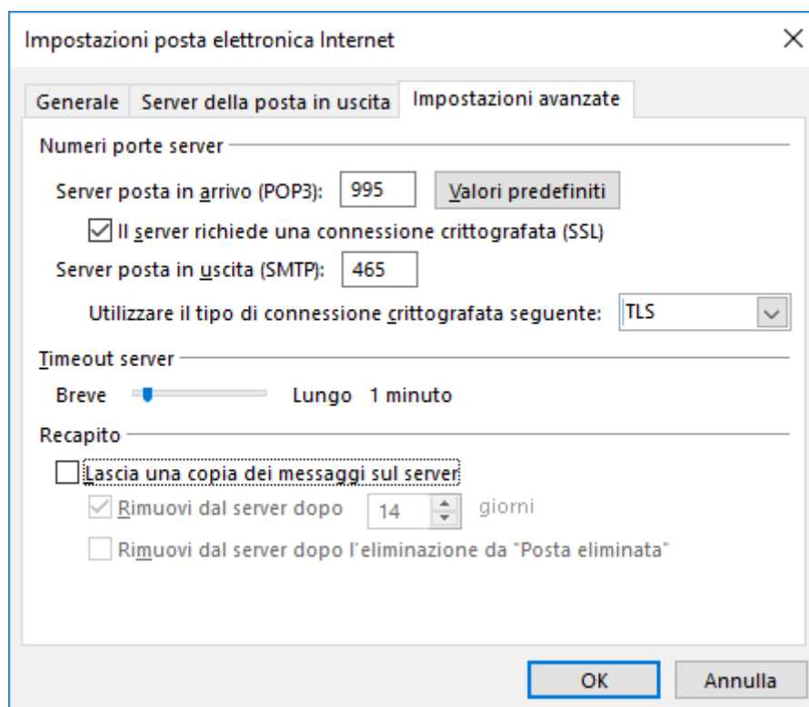
Figura 7: scheda Impostazioni avanzate
